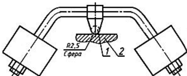
Рисунок 18 - Аппарат для испытания давлением шарика (9.14.2)
