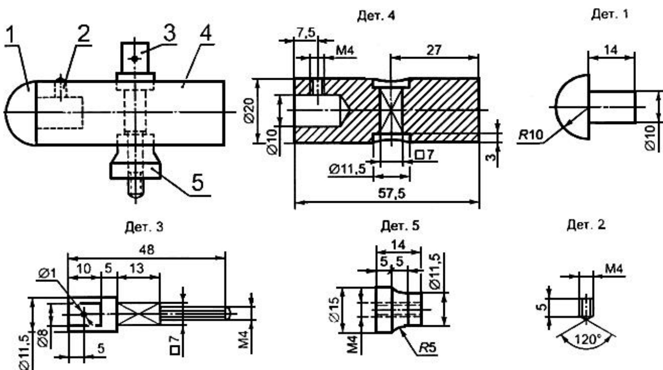
Рисунок 13 - Ударный элемент для маятникового аппарата для испытаний на механический удар (9.12.2.1)
