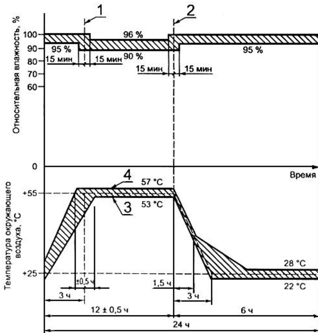
Рисунок 21 - Цикл испытаний на надежность (9.22.1.3)
