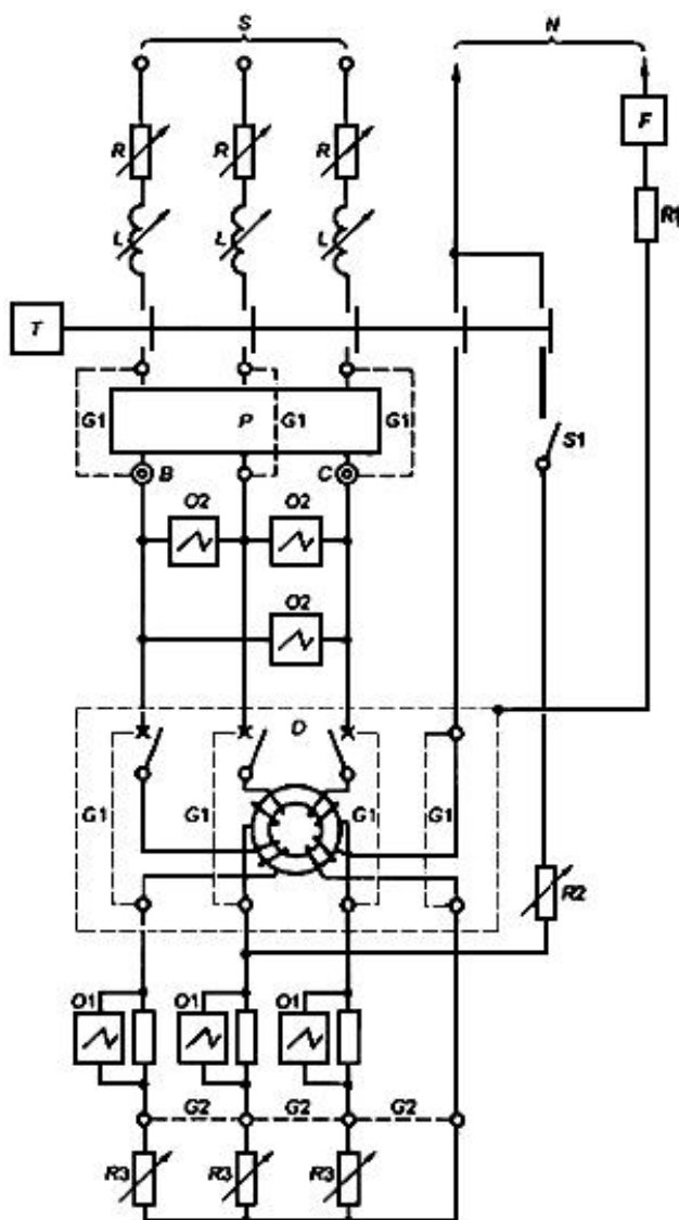
Рисунок 8 - Испытательная цепь для проверки номинальной наибольшей включающей и отключающей способности и координации с ПЗУ трехполюсного ВДТ с четырьмя токовыми путями в трехфазной сети с нейтралью (9.11)
