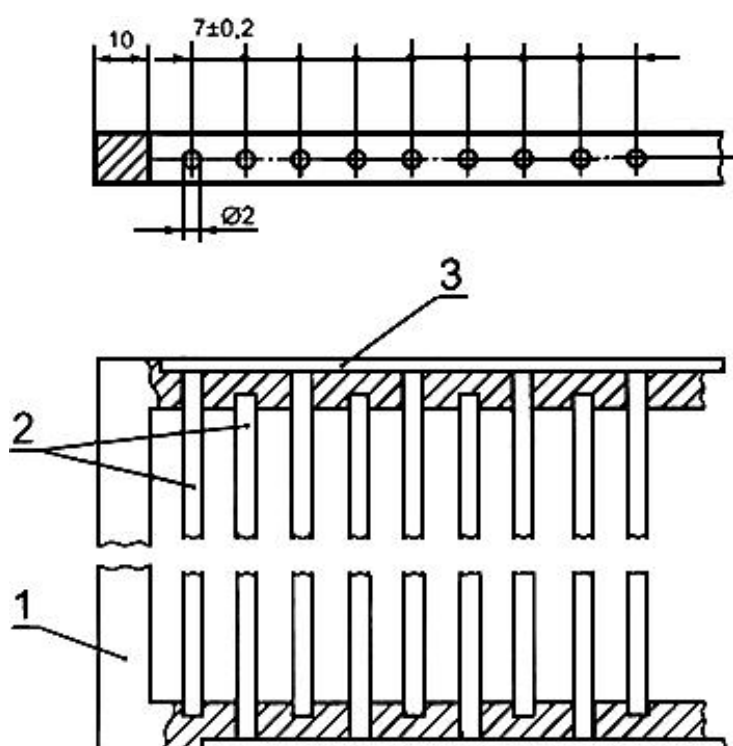
Рисунок С.2 - Сетка
