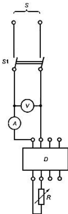
Рисунок 19 - Испытательная цепь для проверки предельной величины сверхтока при однофазной нагрузке трех- или четырехполюсного ВДТ (9.18.2)
