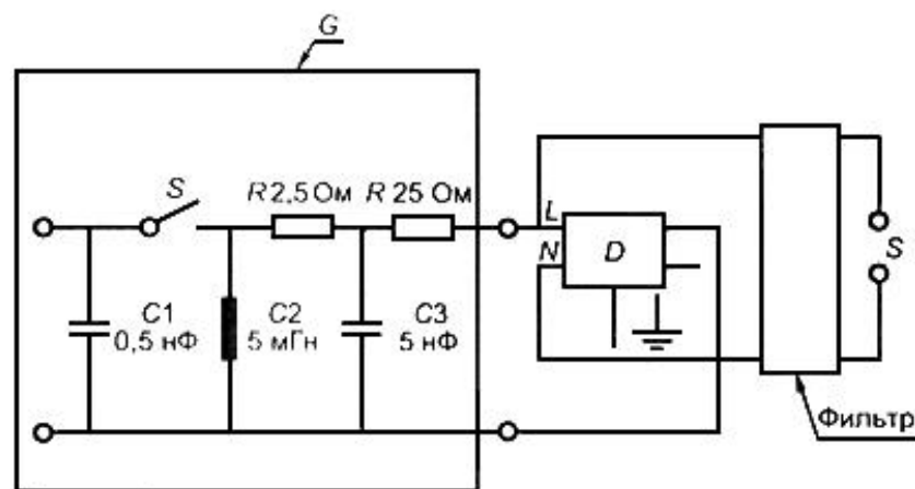
Рисунок 19b - Испытательная цепь для испытания ВДТ звенящей волной
