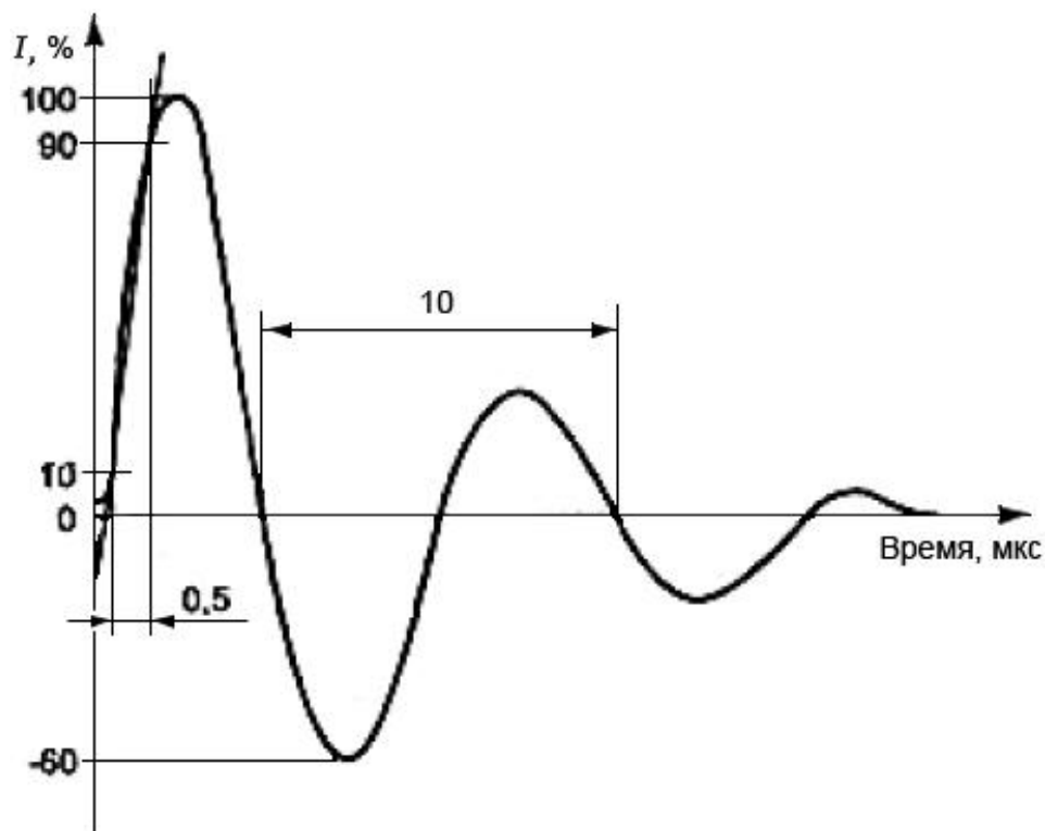
Рисунок 19а - Ток звенящей волны 0,5 мкс/100 кГц
